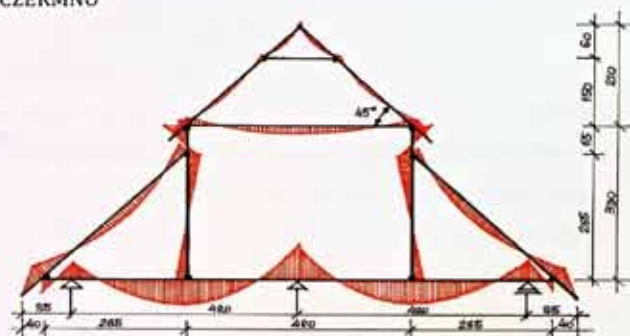
WYKRES MOMENTÓW SIŁ W WIEŻBIE DACHOWEJ
