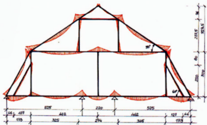
WYKRES MOMENTÓW SIŁ W PRZEKROJACH WIĘZBY DACHOWEJ
