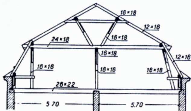
PRZEKRÓJ WIĘZBY DACHOWEJ ( TYP ZE ŚCIANKĄ KOLANKOWĄ )
