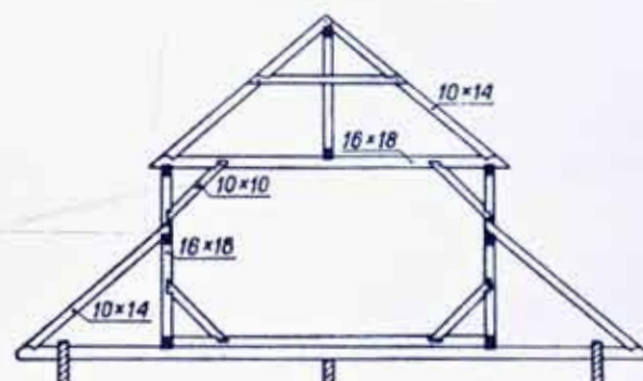
PRZEKRÓJ WIĘZBY DACHOWEJ
