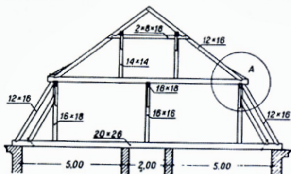
PRZEKRÓJ WIĘZBY DACHOWEJ ( DACH PRZYSTOSOWANY DO RYNNY LEŻĄCEJ NA GZYMSIE )
