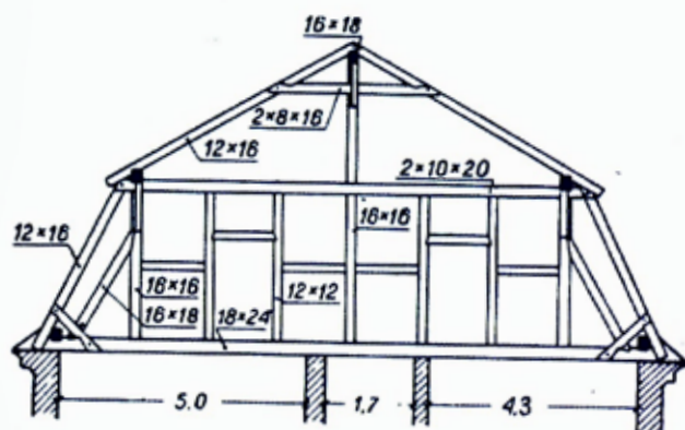
PRZEKRÓJ WIĘZBY DACHOWEJ ( DACH PRZYSTOSOWANY DO RYNNY LEŻĄCEJ ZA GZYMSEM )
