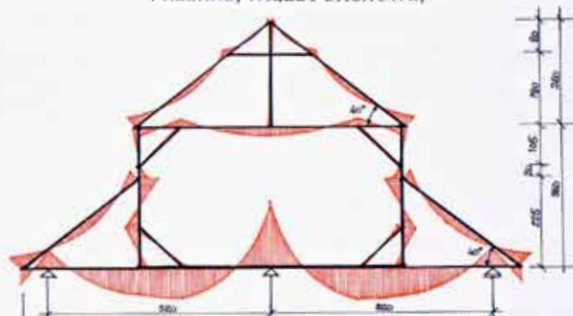
WYKRES MOMENTÓW SIŁ W WIĘZBIE DACHOWEJ
